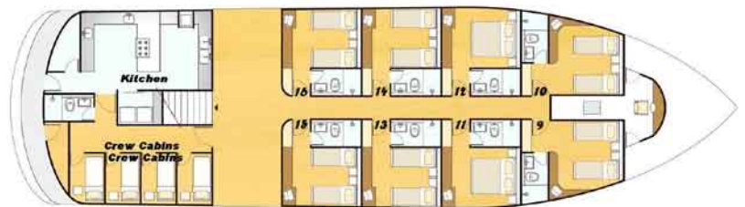
Hauptdeck
